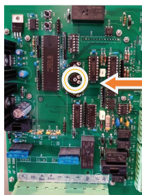
TRIMMER REGOLAZIONE VELOCITÀ
